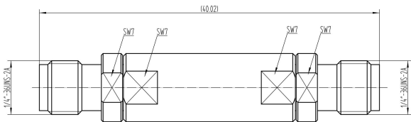
TLME-6G18G-09-FF
